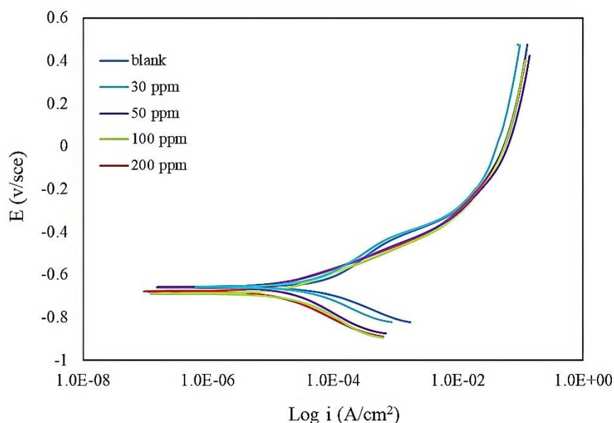
شکل ۶. منحنی های پلاریزاسیون پتانسیودینامیک فولاد کربنی ساده در محیط کلرید سدیم ۳/۵ درصد غیاب و حضور غلظت های مختلف نورتریپتیلین در دمای محیط.
