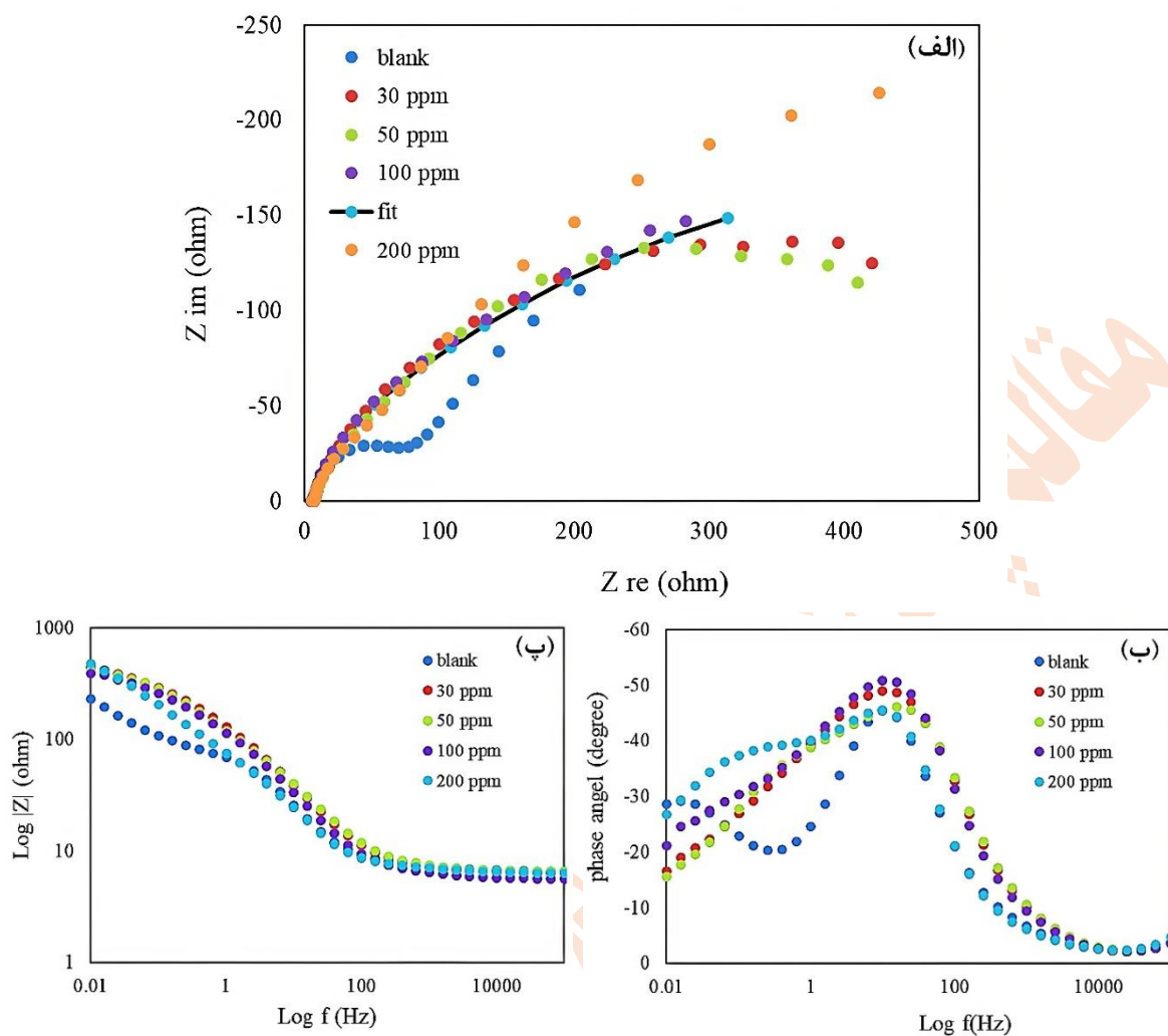
شکل ۷. نمودارهای (الف) نایکوئیست، (ب) بد-فاز و (پ) بد-اندازه امپدانس برای فولاد کربنی در محلول کلرید سدیم ۳/۵ درصد وزنی در حضور و عدم حضور بازدارنده نورتریپتیلین.
