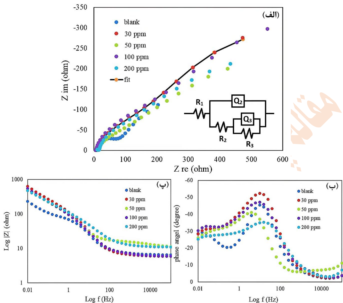
شکل ۳. نمودارهای (الف) نایکوئیست، (ب) بد-فاز، و (پ) بد-اندازه امپدانس برای فولاد کربنی در محلول کلرید سدیم ۳/۵ درصد وزنی در حضور و عدم حضور بازدارنده بیسموت سابسیترات.
