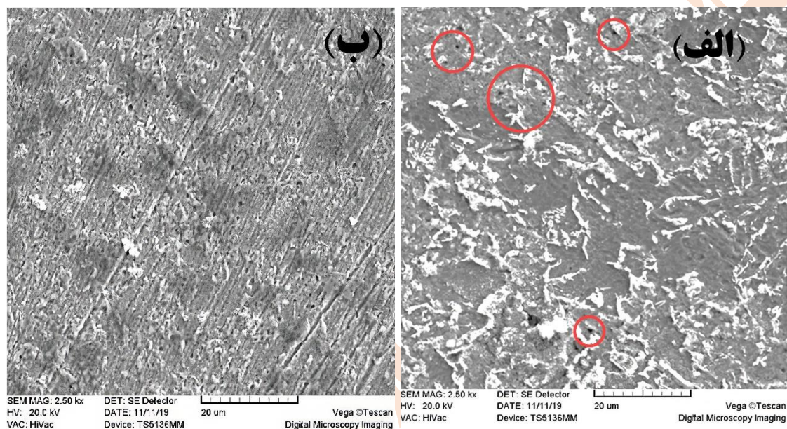
شکل ۴. تصاویر SEM مربوط به نمونه فولاد کربنی پس از ۴۸ ساعت غوطه‌وری در محلول کلرید سدیم (الف) بدون حضور بازدارنده و (ب) در حضور ۳۰ ppm بازدارنده بیسموت ساب‌سیترات.
