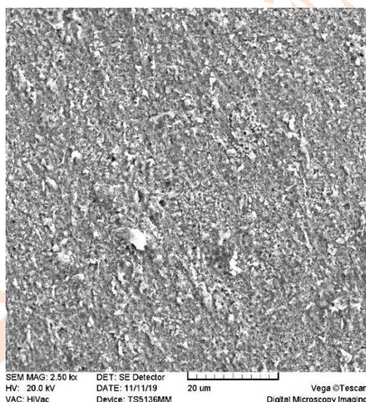
شکل ۸. تصویر SEM مربوط به نمونه فولاد کربنی پس از ۴۸ ساعت غوطه‌وری در محلول کلرید سدیم حاوی ۲۰۰ ppm نورتریپتیلین.
