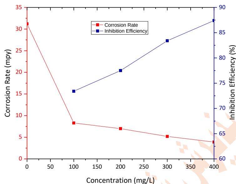
شکل ۱- نمودار تغییرات سرعت خوردگی و درصد بازدارندگی بر حسب غلظت اسانس آویشن شیرازی برای خوردگی فولاد در محلول اسید کلریدریک
