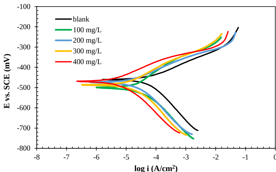
شکل ۴- منحنی پلاریزاسیون نمونه فولادی در محلول اسید کلریدریک حاوی مقادیر مختلف اسانس آویشن شیرازی
