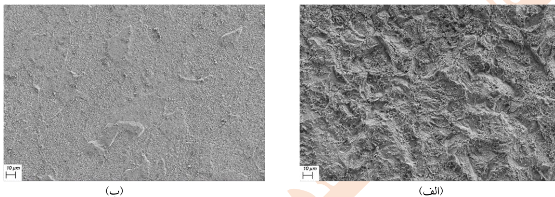
شکل ۶- تصاویر میکروسکوپ الکترونی روبشی از سطح نمونه فولاد در محلول اسید کلریدریک (الف) بدون بازدارنده (ب) حاوی ۴۰۰ mg/L اسانس آویشن شیرازی
