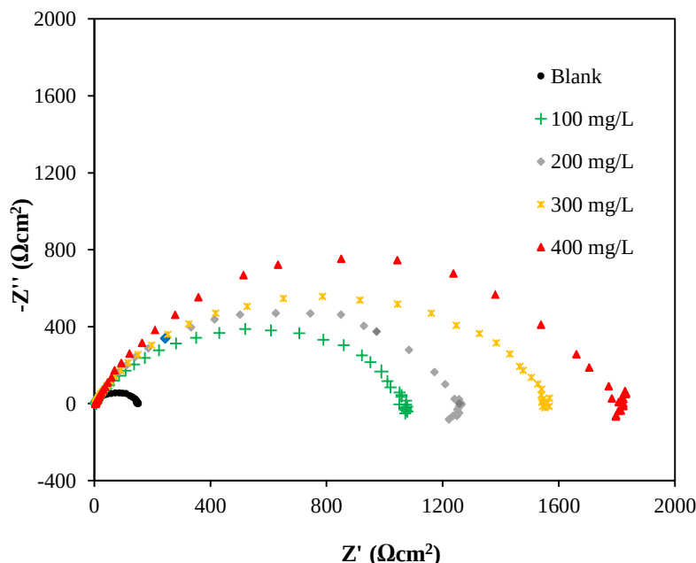
شکل ۲- منحنی نایکوئیست الکتروشیمیایی نمونه فولادی در محلول اسید کلریدریک حاوی مقادیر مختلف اسانس آویش شیرازی
