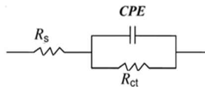
شکل ۳- مدار معادل رندلز
