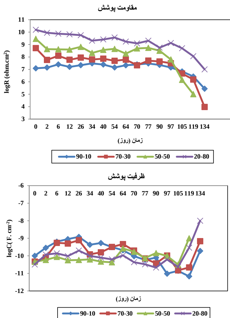
شکل ۸. تغییرات مقاومت و ظرفیت خازنی پوشش‌های ۲۰-۸۰ و ۵۰-۵۰ و ۷۰-۳۰ و ۹۰-۱۰ در طول زمان رطوبت‌دهی
