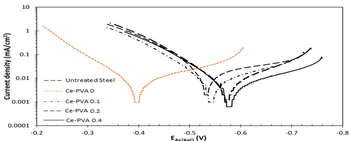
شکل ۴- منحنی‌های پلاریزاسیون برای نمونه‌های فولادی بدون پوشش و پوشش داده شده در حمام پوشش تبدیلی پایه سریم در دمای ۲۵ درجه ی سانتی گراد و pH= ۲/۵ و مدت زمان غوطه‌وری ۱۰ دقیقه برای هر نمونه در غلظت‌های متفاوت از پلی وینیل الکل (PVA) در محلول ۳/۵ درصد وزنی سدیم کلرید (NaCl).
