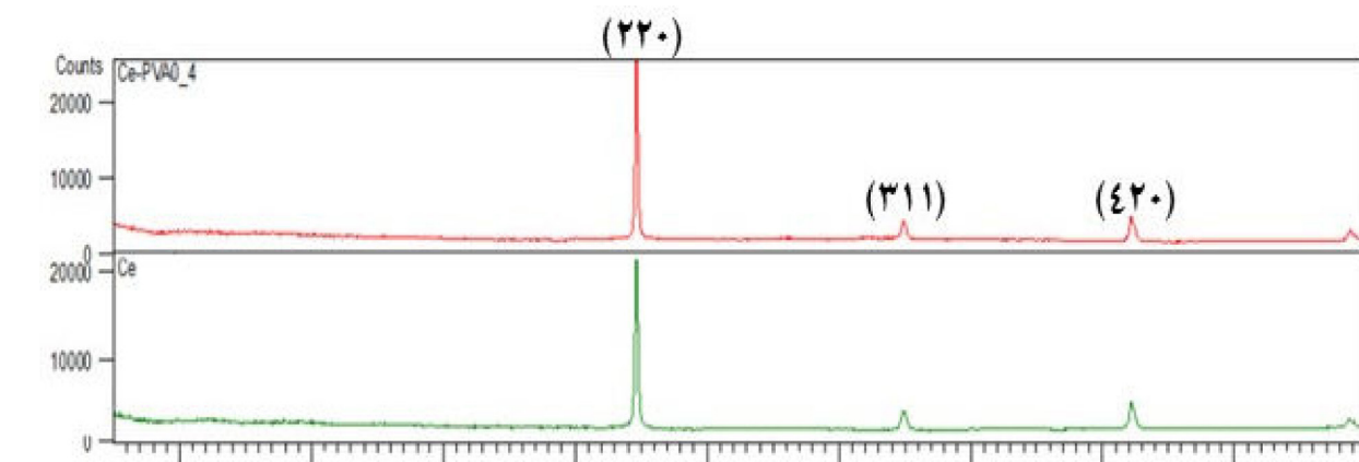
شکل ۶- نتایج آزمون XRD برای نمونه‌های پوشش داده شده در حمام پوشش تبدیلی پایه سربم در حضور PVA (بخش بالایی شکل) و در عدم حضور PVA (بخش پایینی شکل) در حمام.
