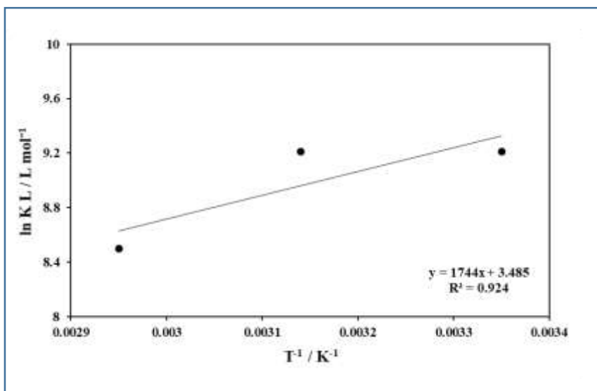
شکل ۱۰ - نمودار وانت - هوف برای جذب بازدارنده روی سطح فولاد X۷۰ در محلول کلریدریک اسید ۱M.
