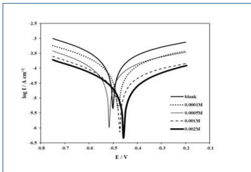
شکل ۲ - منحنی پلاریزاسیون تافل فولاد X۷۰ محلول کلریدریک اسید ۱M در غیاب و حضور بازدارنده با غلظت‌های مختلف در دمای ۲۵ °C سرعت پویش: ۱mV/s.
