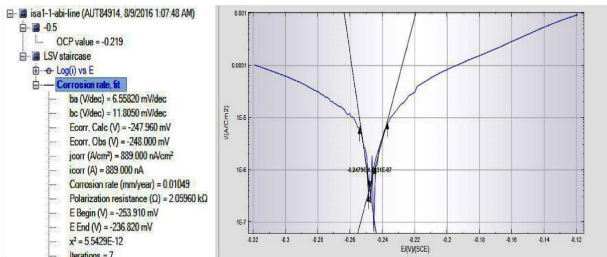
شکل ۲ - نمونه‌ای از اندازه‌گیری پارامترهای آزمون پتانسیودینامیک در محیط برنامه NOVA 1.8 (نمونه‌ی جوشکاری شده با فلز پرکننده ی-ER۳۰۹L و بدون پیش گرم (نمونه S۴))
