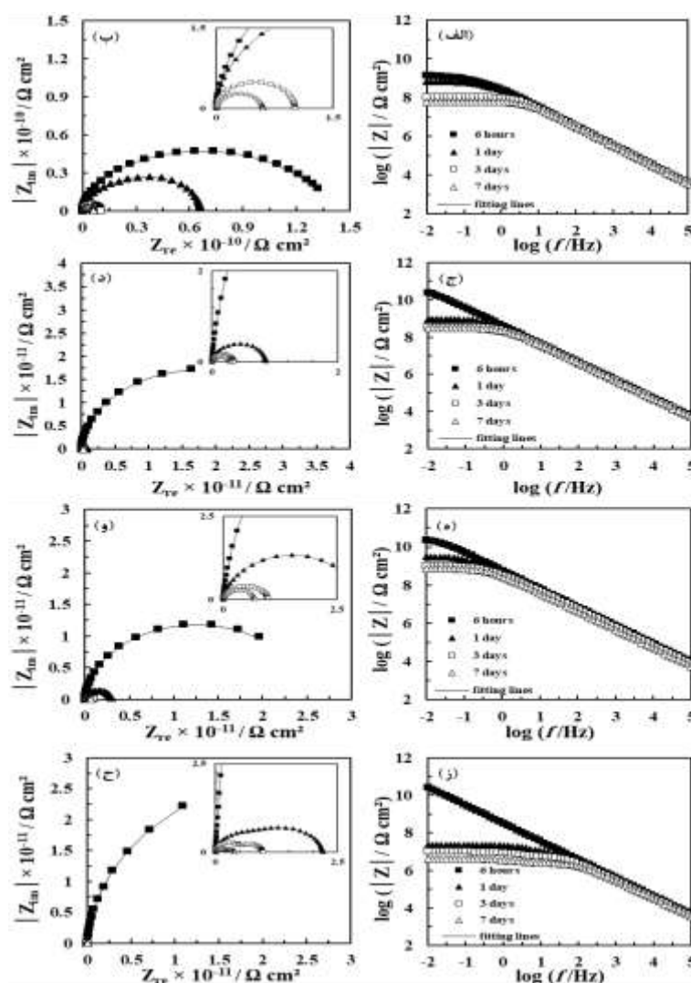
شکل ۱ - نمودارهای نایکوئیست و بُد پوشش‌های پلی‌یورتان ساخته شده با نسبت‌های مختلف NCO/OH: (الف، ب) NCO/OH = 1 و (ج، د) NCO/OH = 1.1، (ه، و) NCO/OH = 1.2 و (ز، ح) NCO/OH = 1.3 غوطه‌ور شده در محلول اسید سولفوریک یک مولار در زمان‌های مختلف و در دمای محیط.
