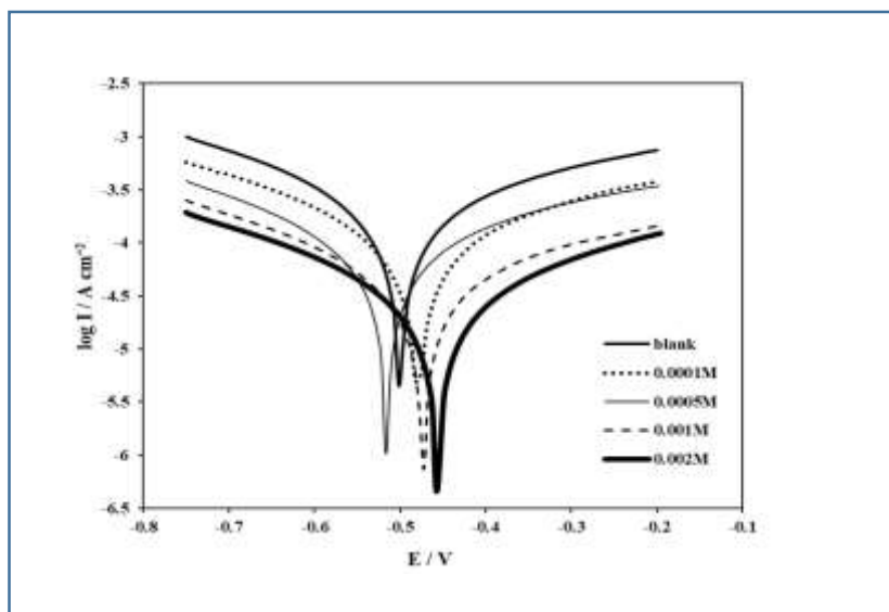
شکل ۲ - منحنی پلاریزاسیون تافل فولاد X۷۰ محلول کلریدریک اسید ۱M در غیاب و حضور بازدارنده با غلظت های مختلف در دمای ۲۵ °C سرعت پویش: ۱mV/s.
