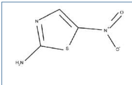
شکل ۱ - ساختار شیمیایی ۲-آمینو - ۵- نیترو تیا زول.
