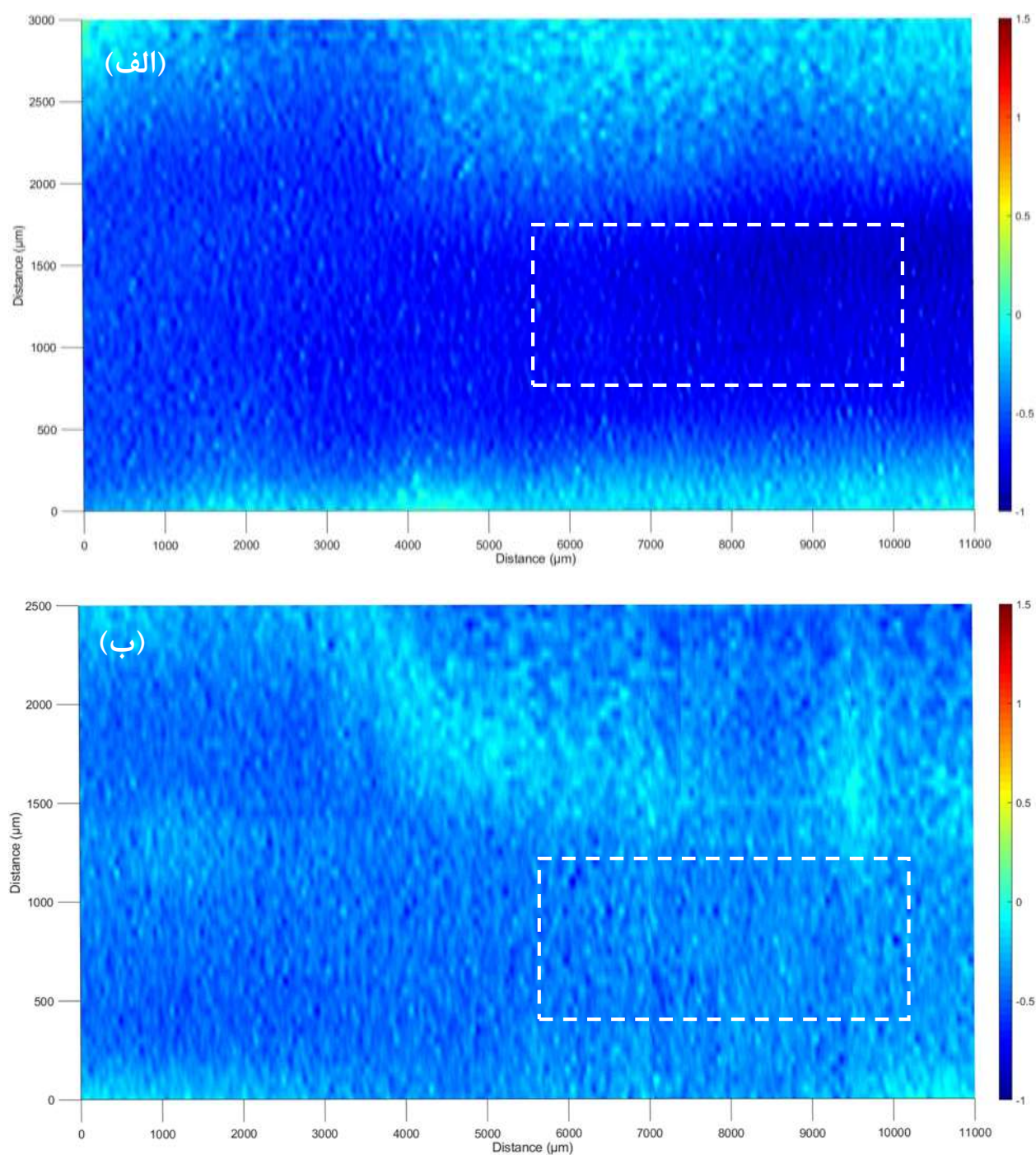
شکل ۳- توزیع پتانسیل سطحی (بر حسب SCE) روی سطح مقطع عرضی نمونه‌های آلومینیمی جوشکاری شده با روش PFSSW با سرعت چرخش ابزار ۲۵۰۰ دور بر دقیقه: (الف) قبل از غوطه‌وری و (ب) بعد از ۲۰ ساعت غوطه‌وری در محلول کلرید سدیم ۳/۵ درصد وزنی در دمای اتاق و شرایط ساکن.
