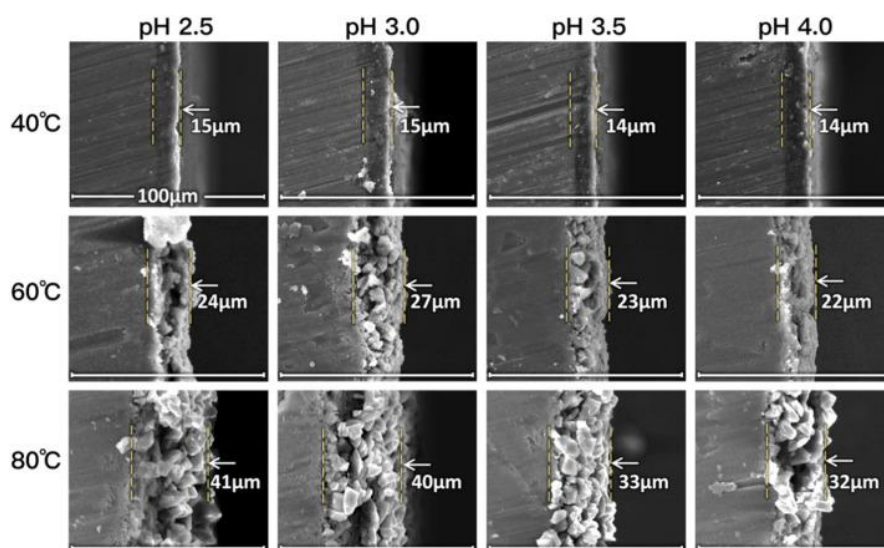
شکل ۶ - مورفولوژی سطح مقطع نمونه‌های پوشش داده شده در دمای ۴۰، ۶۰ و ۸۰ درجه سانتی‌گراد با مقادیر pH مختلف [۸]
