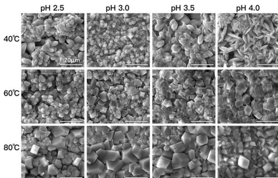
شکل ۵ - مورفولوژی سطح نمونه‌های پوشش داده شده در دمای ۴۰، ۶۰ و ۸۰ درجه سانتی‌گراد با مقادیر pH مختلف [۸]
