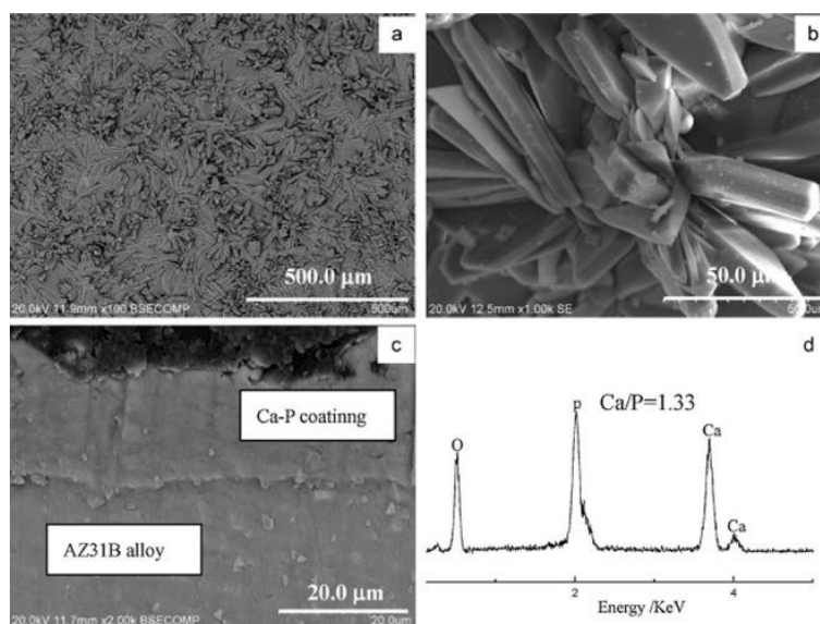
شکل ۱ - مورفولوژی سطح و مقطع نمونه آلیاژ AZ31B با پوشش Ca-P: (a) سطح (b) بزرگ‌نمایی بالا، (c) مقطع، (d) آنالیز EDS روی سطح [۱]
