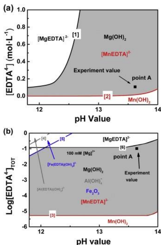
شکل ۱۳ - نمودار مساحت غالب با (a) محاسبه ترمودینامیکی و (b) محاسبه شده از طریق نرم‌افزار مدوزا. خط [۱] و [۲] محاسبات ترمودینامیکی برای گونه‌های حاوی منیزیم و منگنز با استفاده از معادله نرنست بودند؛ خط [۳] [۴] و [۵] محاسبات ترمودینامیکی برای گونه‌های حاوی Mn^{2+} ، Al^{3+} و Fe^{3+} با استفاده از Hydro بودند. نرم‌افزار مدوزا در مجموع ۱۰ میکرومولار. خط [۶] محاسبات ترمودینامیکی برای گونه‌های حاوی Mg^{2+} با استفاده از نرم‌افزار Hydro-Medusa در مجموع ۱۰۰ میلی‌مولار بود [۹].
