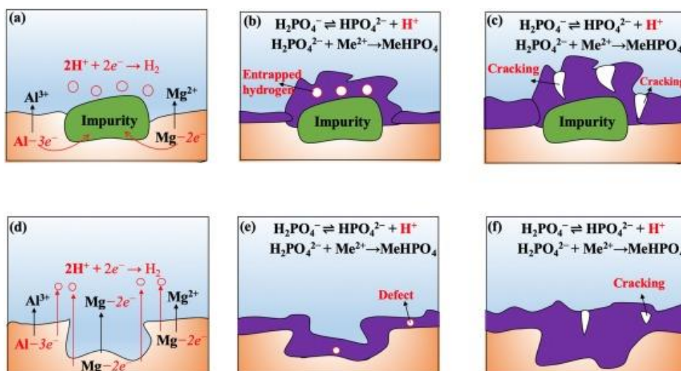
شکل ۱۶ - تصویر شماتیک مکانیسم تشکیل Mn-PCC : (a-c) PCC و (d-b) SP-Mn-PCC [۹]
