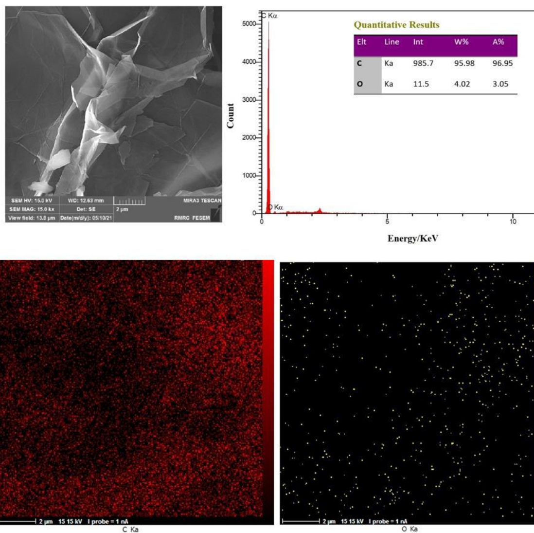
شکل ۳ - آنالیز SEM/MAPPING EDX از نمونه MLGO
