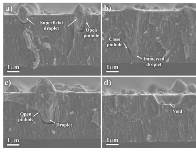
شکل ۱ - مقطع معمولی و ویژگی‌های عیوب به‌دست آمده در پوشش‌های CrN مورد مطالعه: (a) قطرات سطحی با حفره باز، (b) قطره داخلی با منافذ سوزنی بسته، (c) قطره بزرگ با برآمدگی زیاد و منافذ باز، و (d) حفره باز راه‌حلی برای حذف قطرات در پوشش
